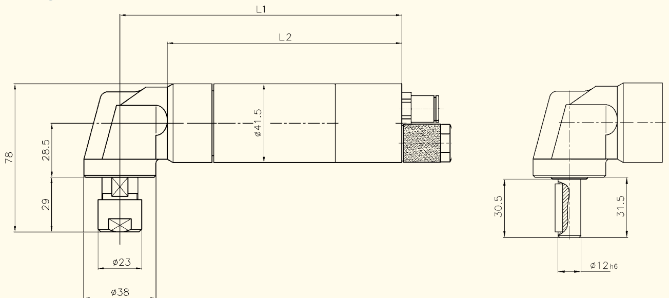
Abmessungen (mm)
